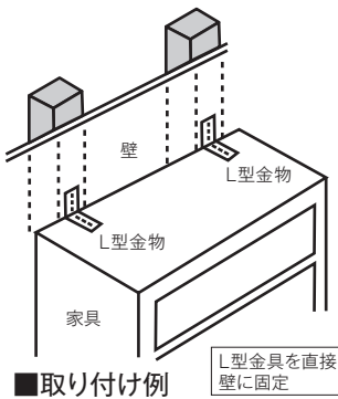
■取り付け例
