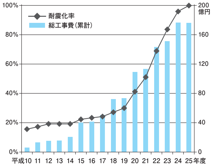
■小・中学校の耐震化率と総工事費の推移
