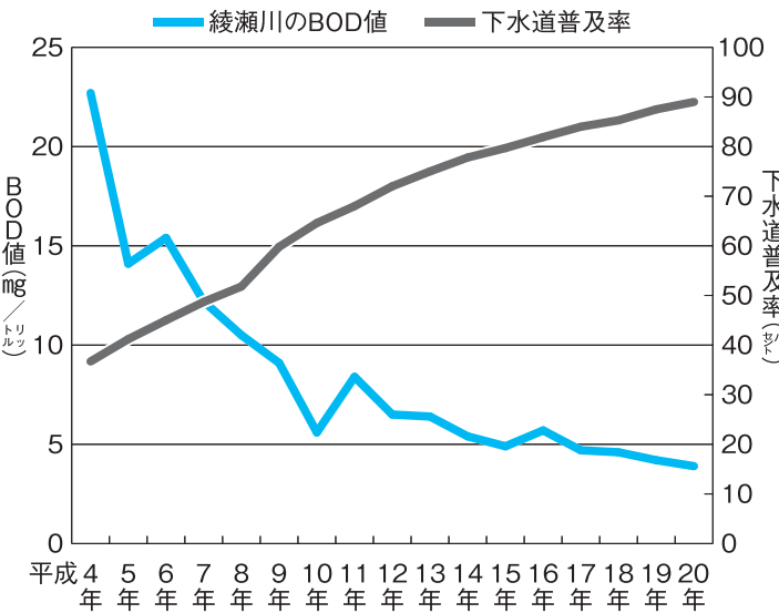
■下水道普及率と水質改善の推移
