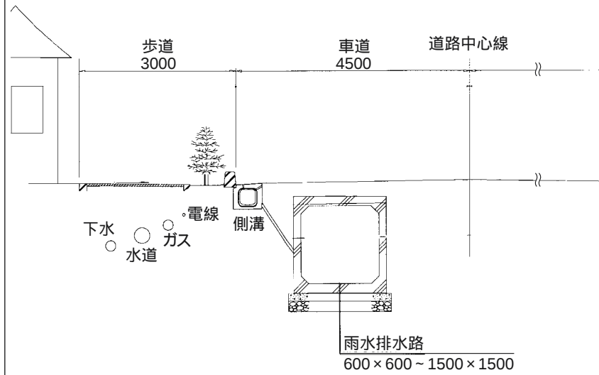
■図2 瀬崎東町線の構造
