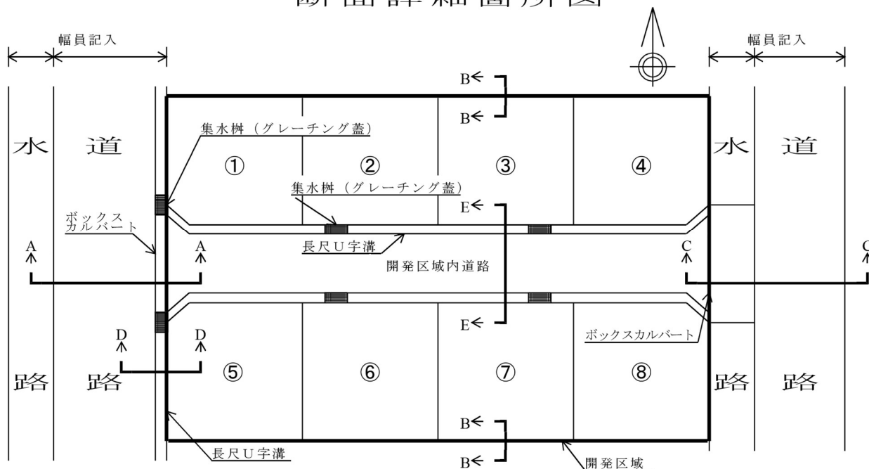
断面詳細箇所図
