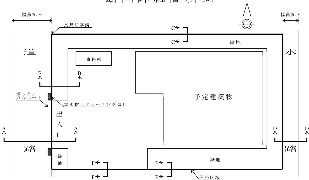
断面詳細箇所図
