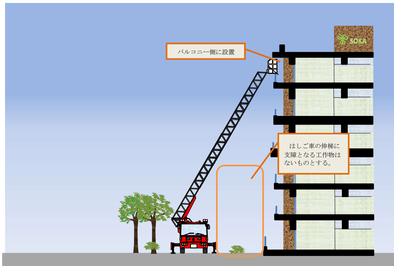
立面図
