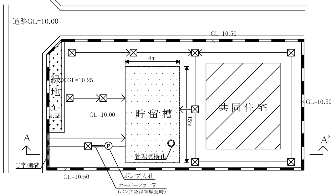
雨水流出抑制施設平面図 (S=Free)
