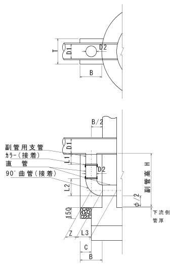
副管設置図
