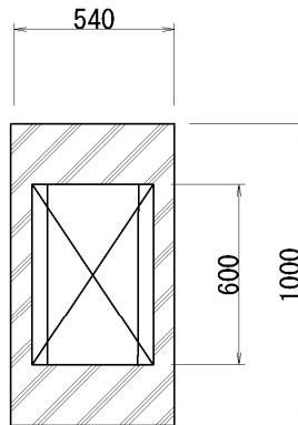
平面図
