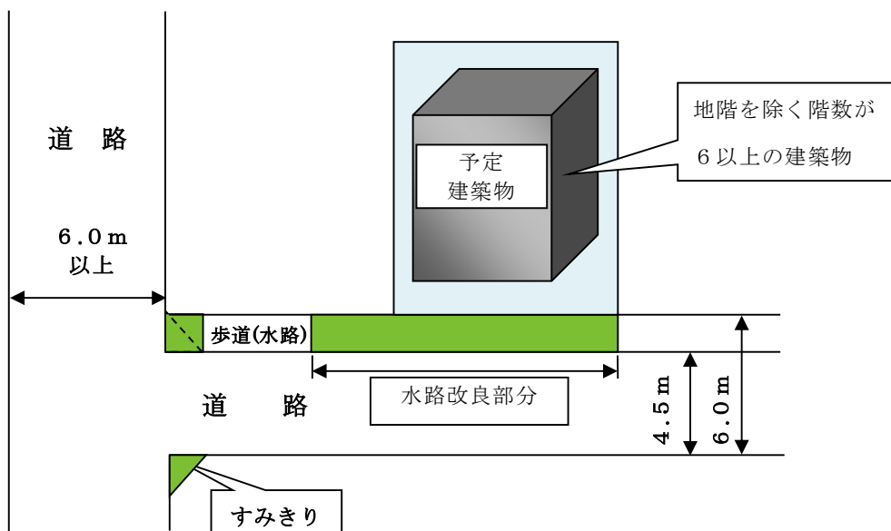
中高層建築物の整備要件参考図
