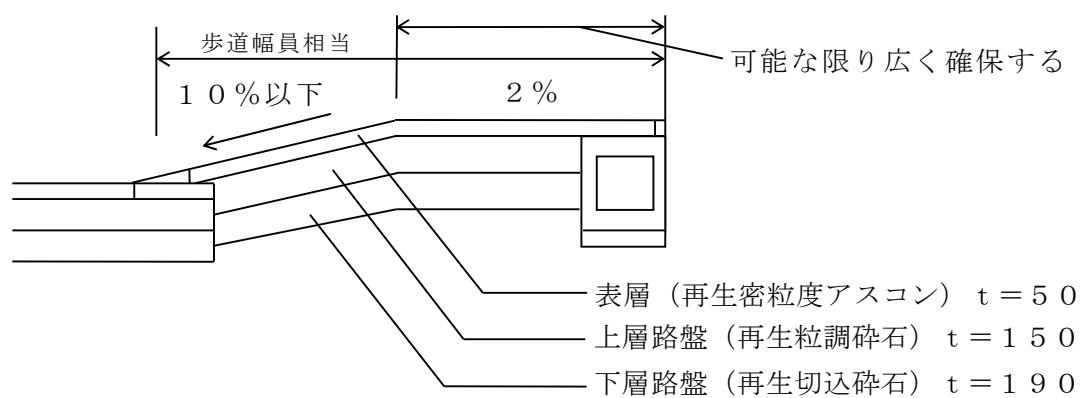
[B - B 断面]
