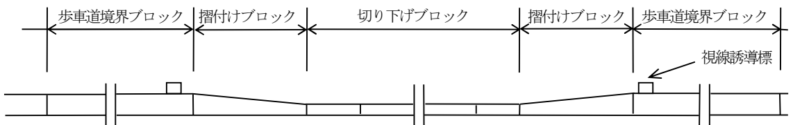
〔A-A 断面〕
