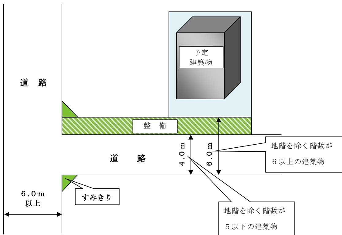
中高層建築物の整備要件参考図
