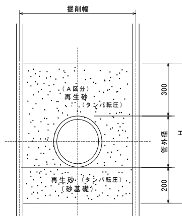
管基礎標準図
