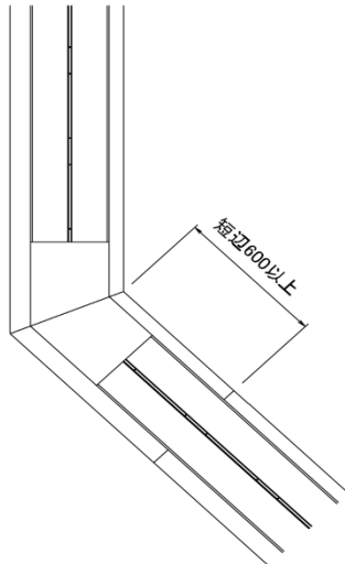
[側溝配置例]
