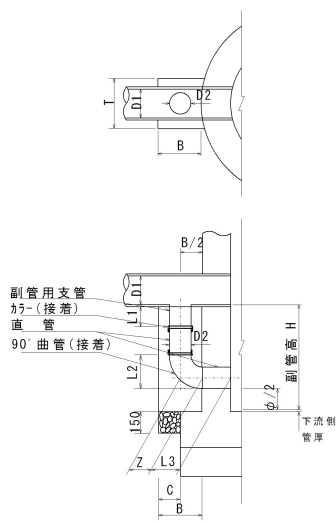
副管設置図
