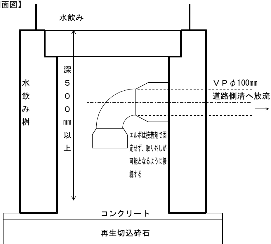
【側面図】
