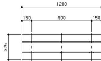
平面図 S=1/20
