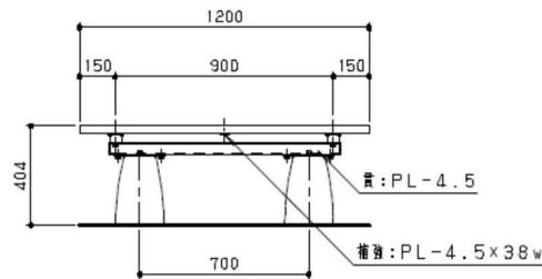
立面図 S=1/20
