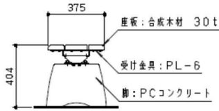
断面図 S=1/20
