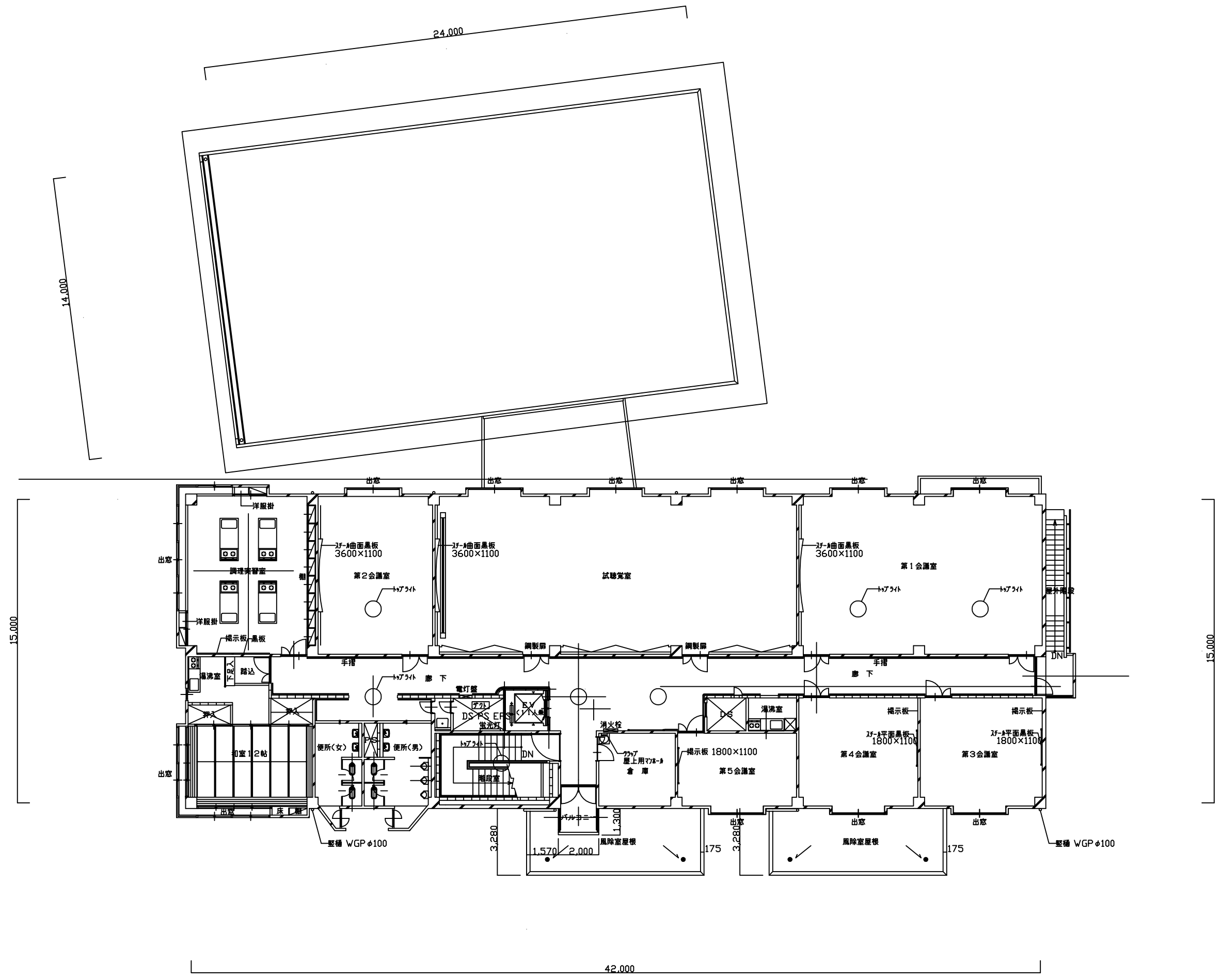
2 階 平 面 図 勤労福祉会館
