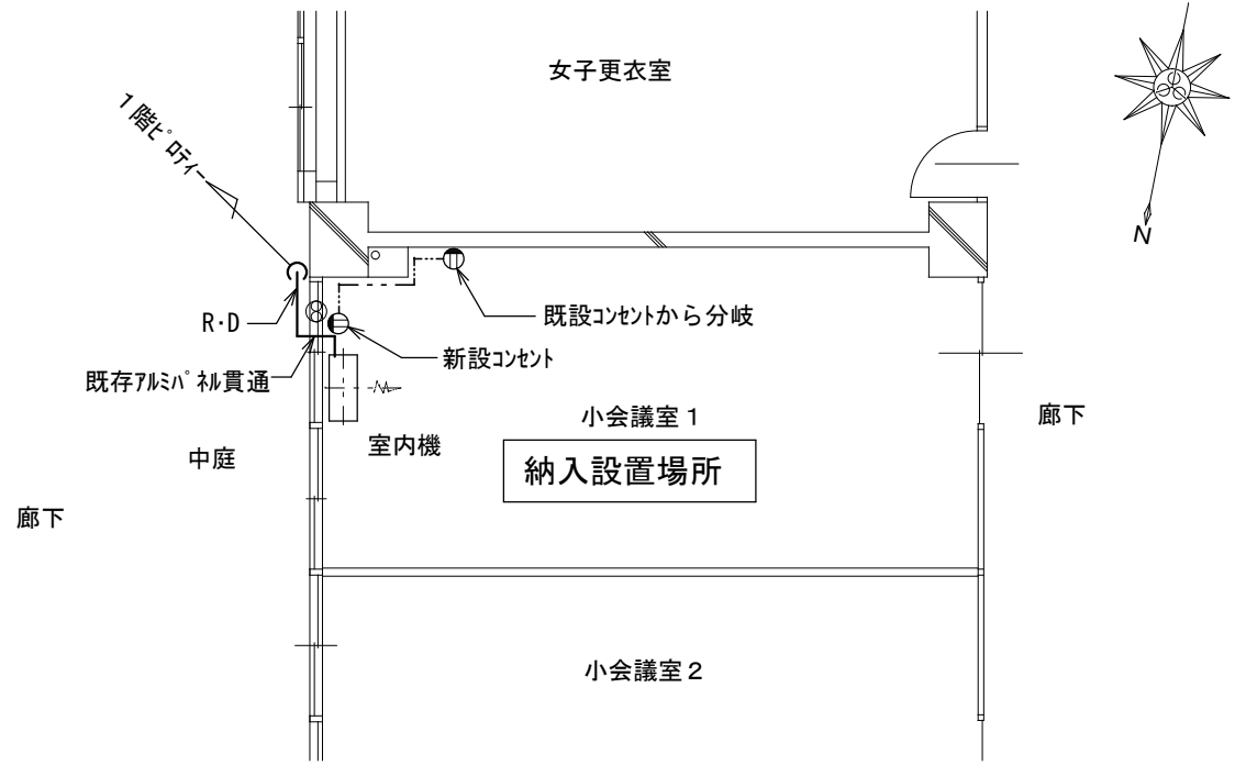
2階平面図 1/100
