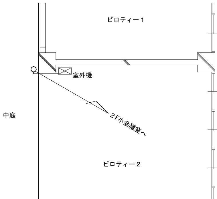
1階平面図 1/100
