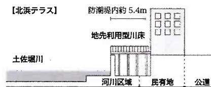
図-2 北浜テラスの断面図
