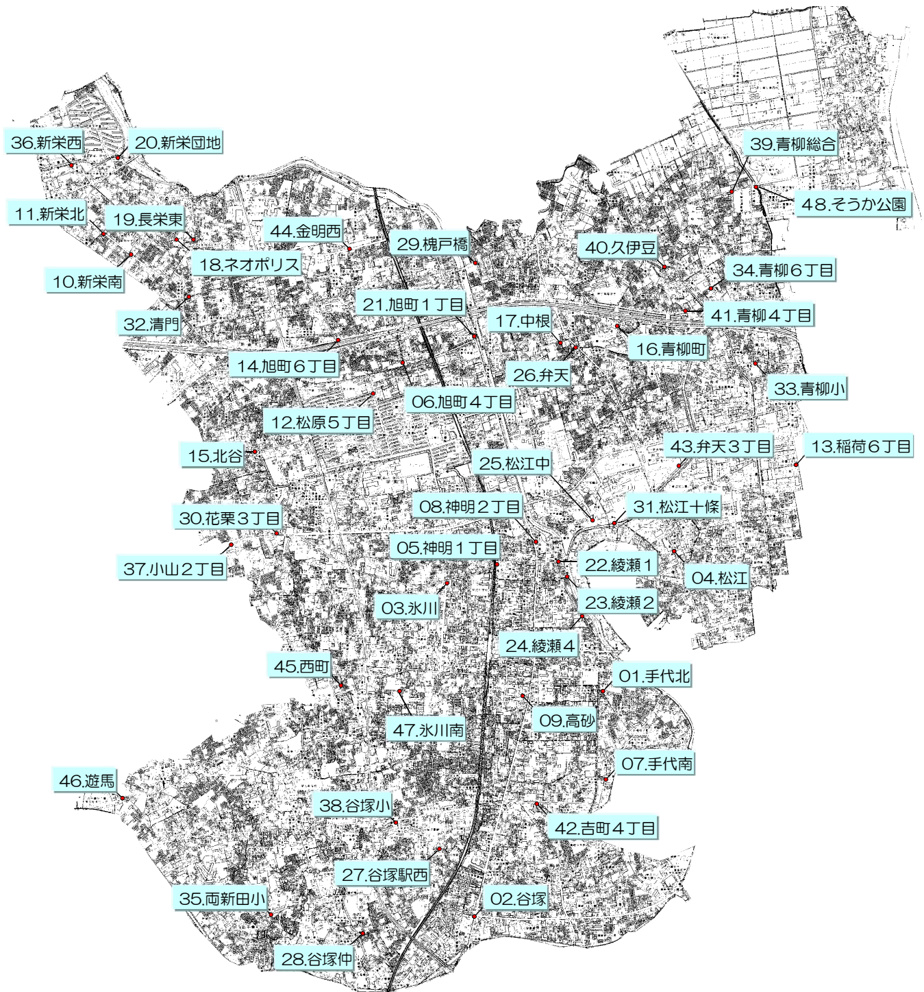
【参考5】汚水マンホールポンプ（48機場）位置図
