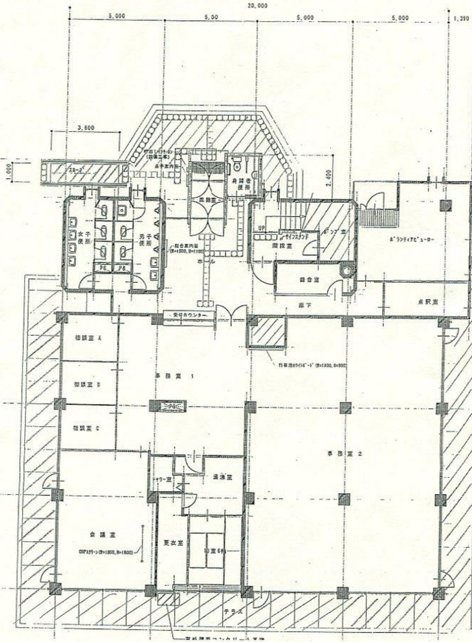
1 階 平 面 図 1:100
